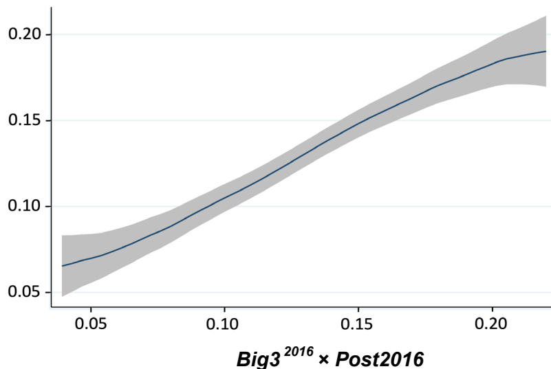
Fig. 4. Kernel Estimation
